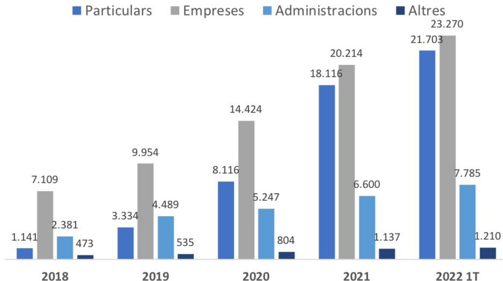
Evolució de la potència instal·lada a Balears per tipus de consumidor (kW)
