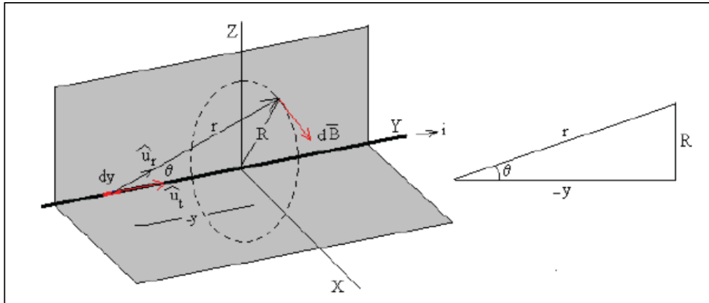
Imagen 4. Campo electromagnético generado por un conductor rectilíneo
