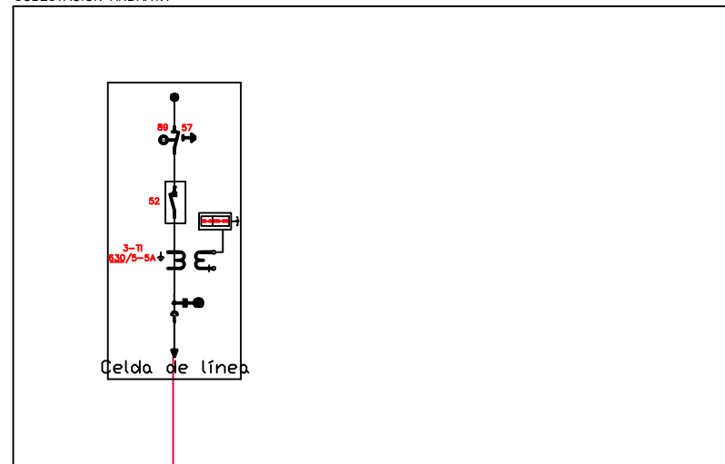
SUBESTACIÓN "ANDRATX"
