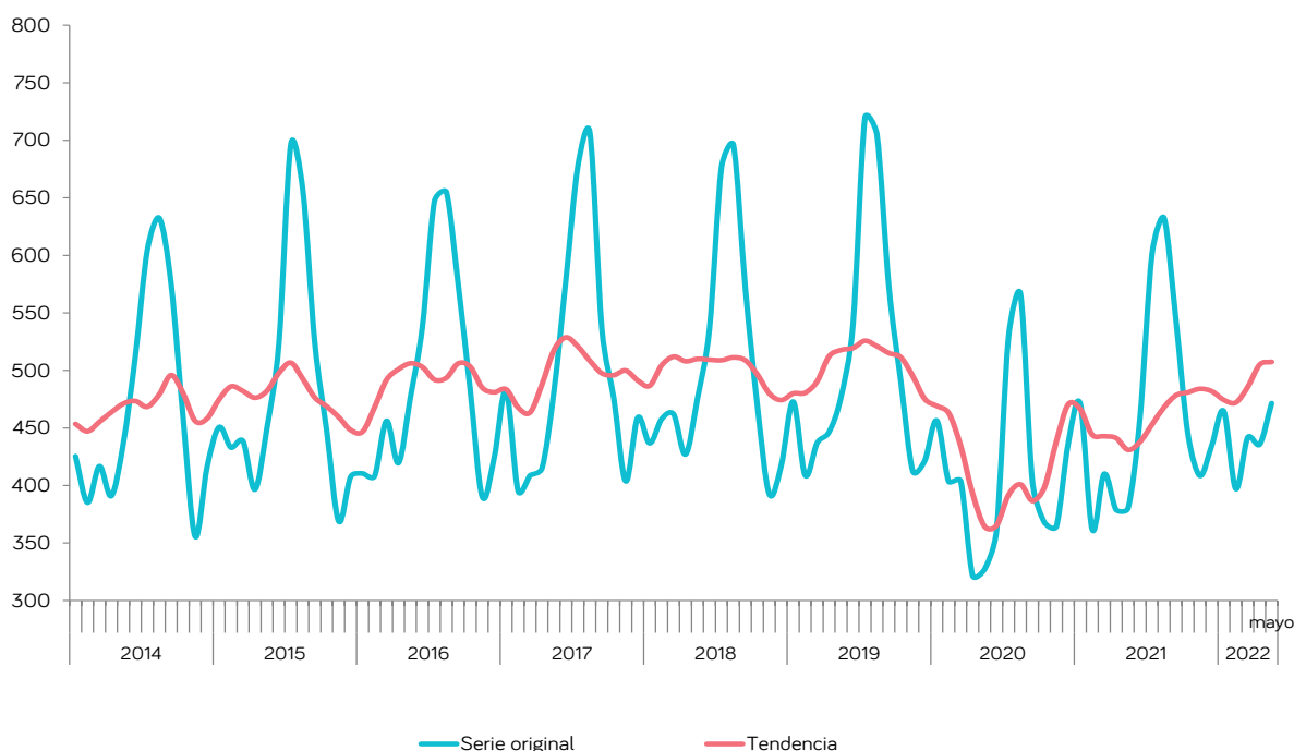
Gráfico 8. Energía eléctrica mensual demandada en las Islas Baleares (GWh)
