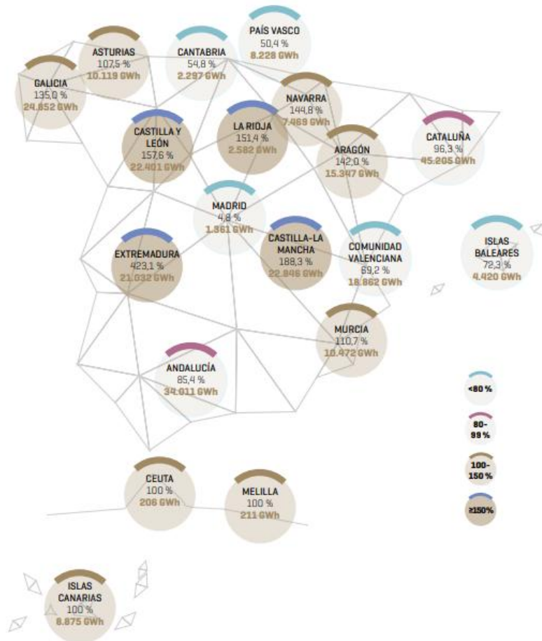
Il·lustració 5: Ràtio generació elèctrica/demanda (%) i generació elèctrica (GWh) en el 2019 per comunitat autònoma. Font: REE- El sistema elèctric espanyol I 2019 15
