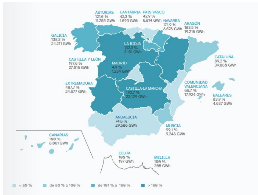
Il·lustració 7: Ràtio generació elèctrica/demanda (%) i generació elèctrica (GWh) en el 2021 per comunitat autònoma. Font: REE- El sistema elèctric espanyol 2021 17 .
