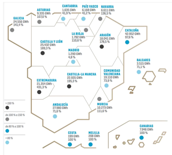
Il·lustració 6: Ràtio generació elèctrica/demanda (%) i generació elèctrica (GWh) en el 2020 per comunitat autònoma. Font: REE- El sistema elèctric espanyol 2020 16 .
