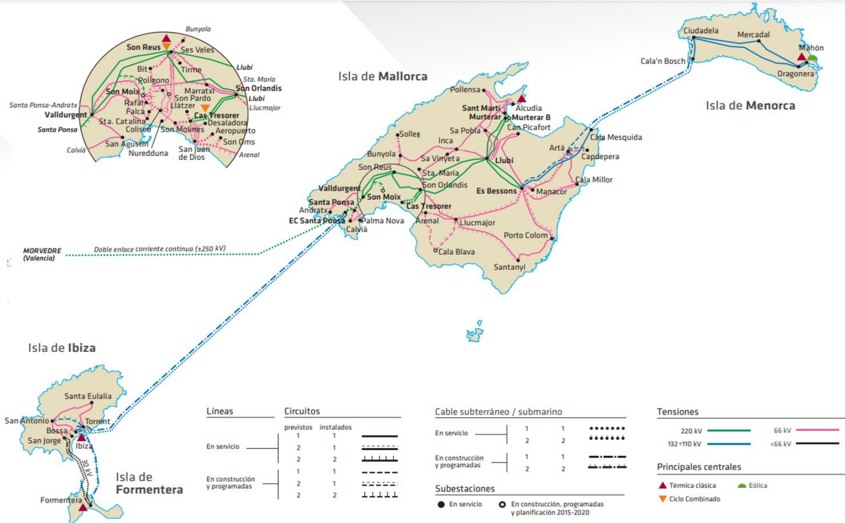
Il·lustració 12: Xarxa de transport balear. Font: REE.
