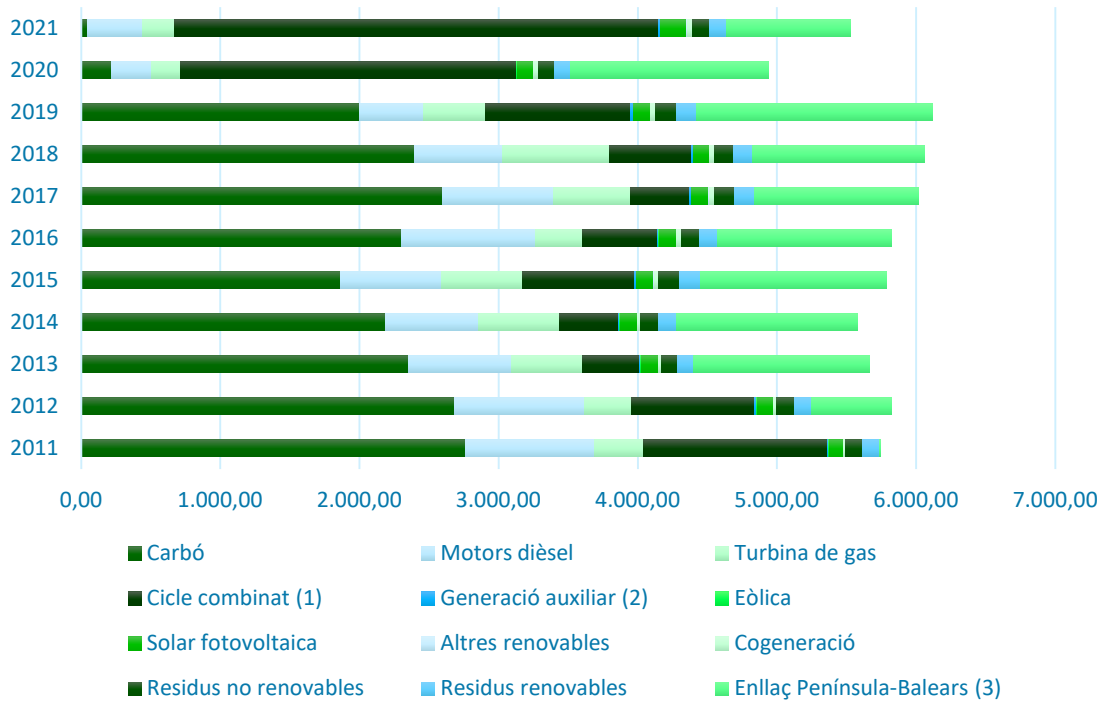
Gràfic 19: Evulsió de la cobertura de la demanda de les Illes Balears (GWh). Font: REE.
