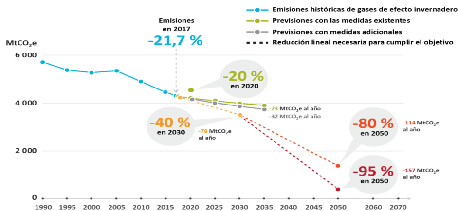
Il·lustració 1: Emissions de GEI de la UE. Font: Tribunal de comptes europeu 3 .
