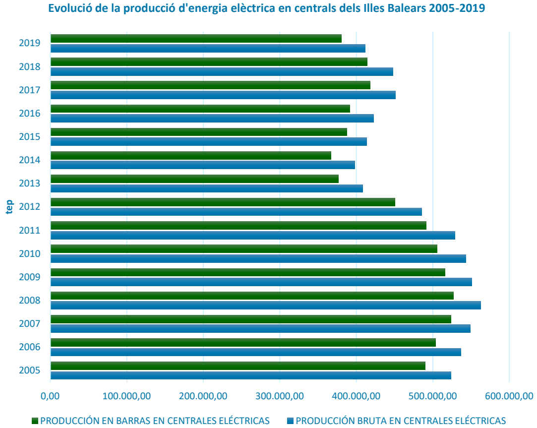
Gràfic 11: Evolució de la producció d'energia elèctrica en centrals de les Illes Balears 2005-2019. Elaboració pròpia. Font: Direcció General d'Energia i Canvi Climàtic > Portal energètic.
