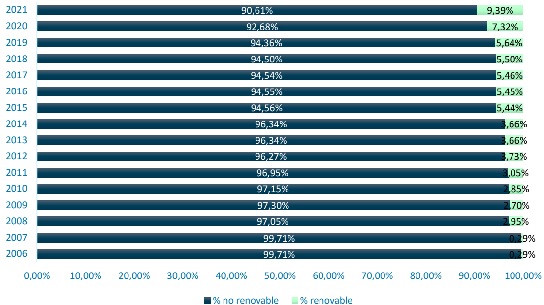
Gràfic 16: Evolució de la generació renovable i no renovable en el sistema balear. Elaboració pròpia. Font REE i CNMC.
